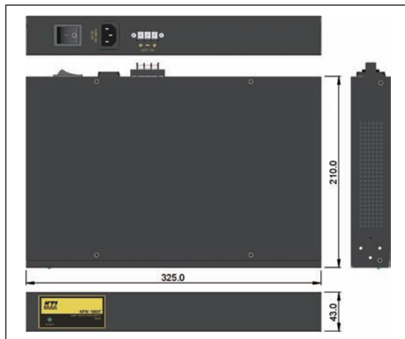
Dimensions
